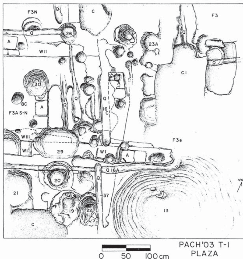
Fig. 6 – Plano 2 de la Trincher 1 en la Plaza de los Peregrinos señalando arquitectura y rasgos de la parte media del Periodo de Intermedio Tardío (Ychsma Medio). Dibujado por Izumi Shimada y César Samillán.
